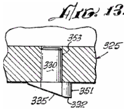
Fig.13 es una vista fragmentaria, tomada en la línea 13---13 en Fig.12
