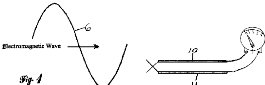
Fig.1 muestra por qué es así. La onda electromagnética de paso 6 genera una carga eléctrica alterna en el cable 10, sintonizada en la frecuencia de la onda para cerrar el circuito para que circule la carga inducida, hemos añadido un segundo cable 11, pero si conectan los extremos de los cables, la onda electromagnética 6 induce una carga en el segundo cable exactamente igual que en el primer cable, y ninguna corriente fluirá. Cualquier intento de circular la carga inducida en alambre 10 está bloqueada por un cargo de oposición igual en 11.
