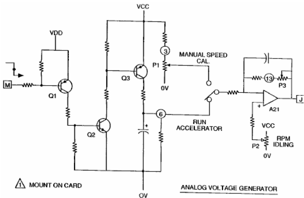
Fig.3 muestra un generador de voltaje análogo.
