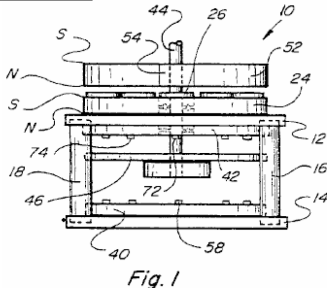
Fig.1 es una vista lateral del dispositivo impulsado de un magnetically construido según la invención presente.
